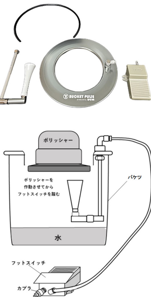
全体図
