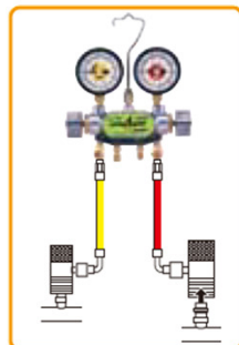
ゲージマニホールド接続時
