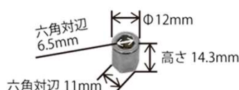
H11ビットアダプター
