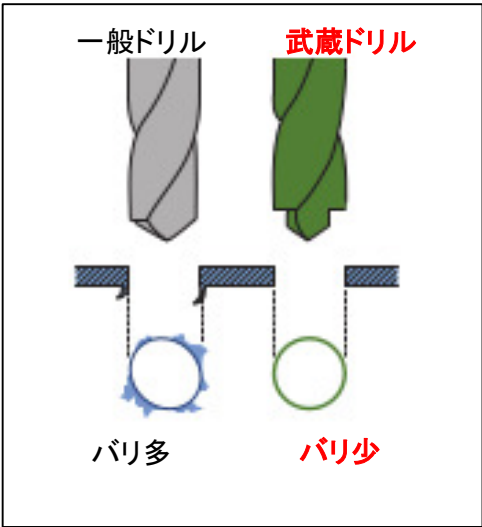
穴あけ加工後の断面
